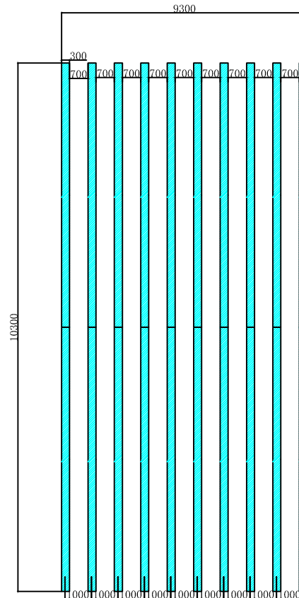
混凝土基础俯视图 总宽度9300mm，总长10300mm
